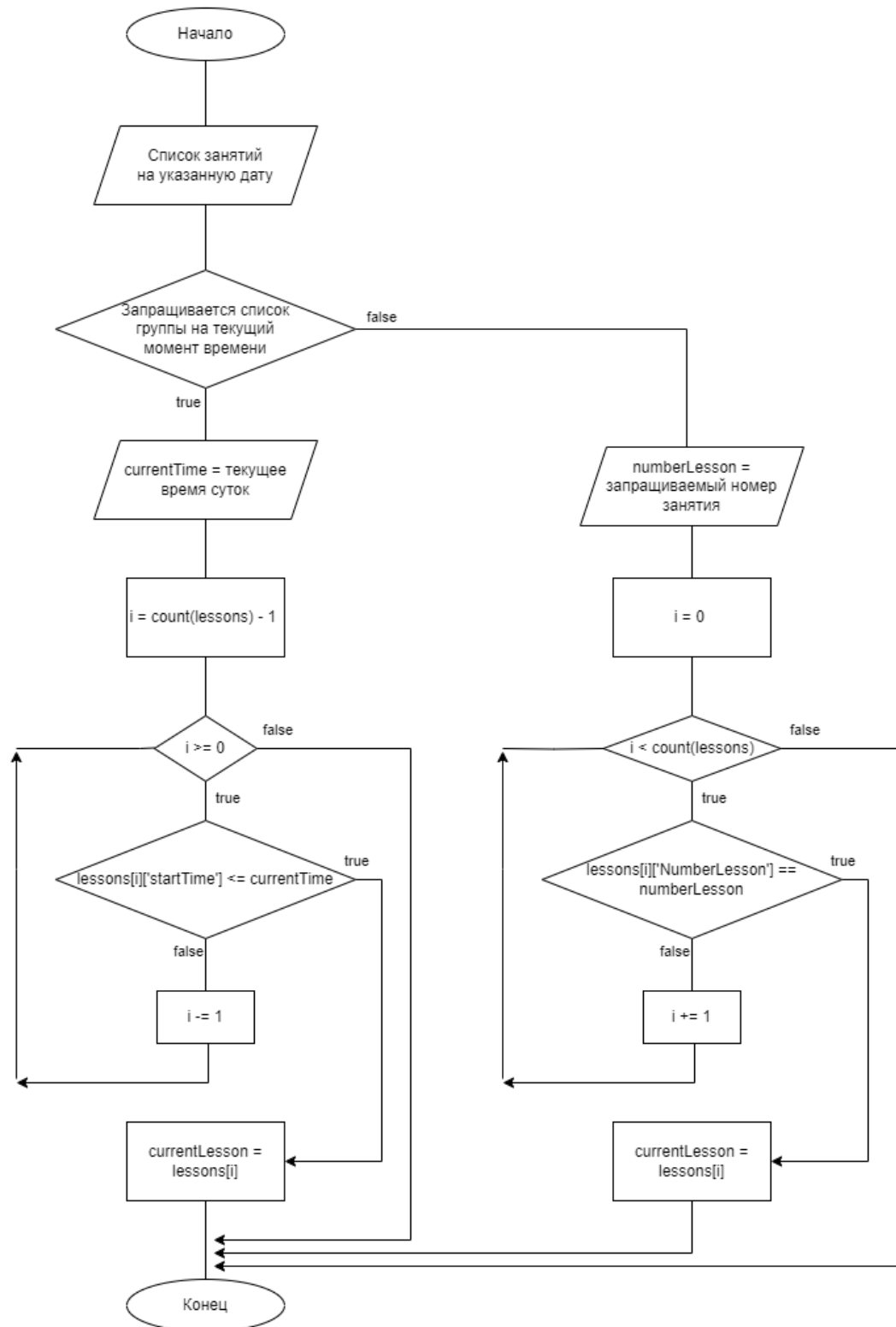
Рисунок 3.4.2 – Алгоритм поиска нужного занятия на текущий момент времени, либо по указанному номеру
