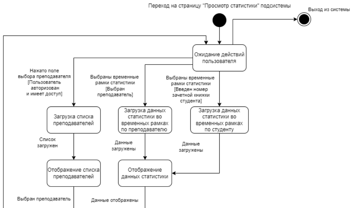
Рисунок 2.2.3 - Множество состояний и переходов страницы «Статистика»
